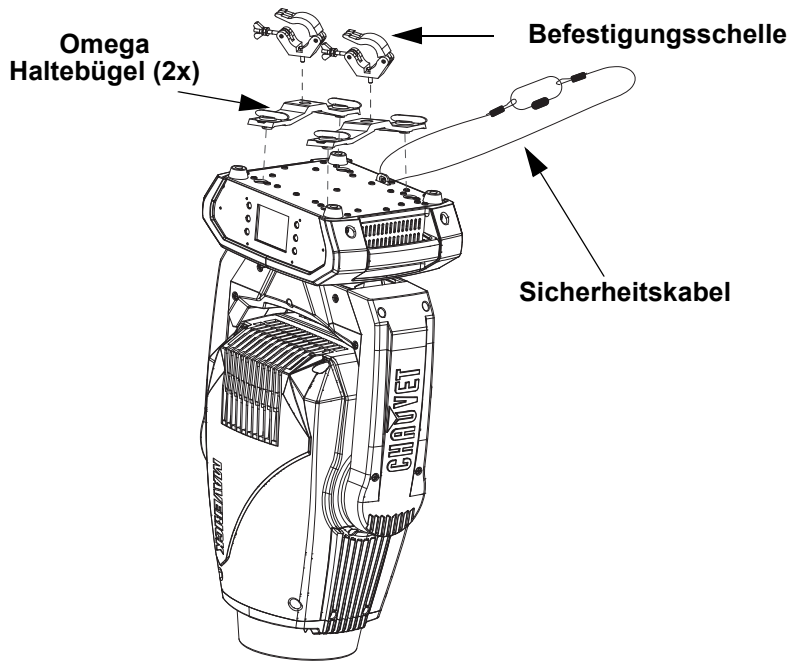
Montage über Kopf
