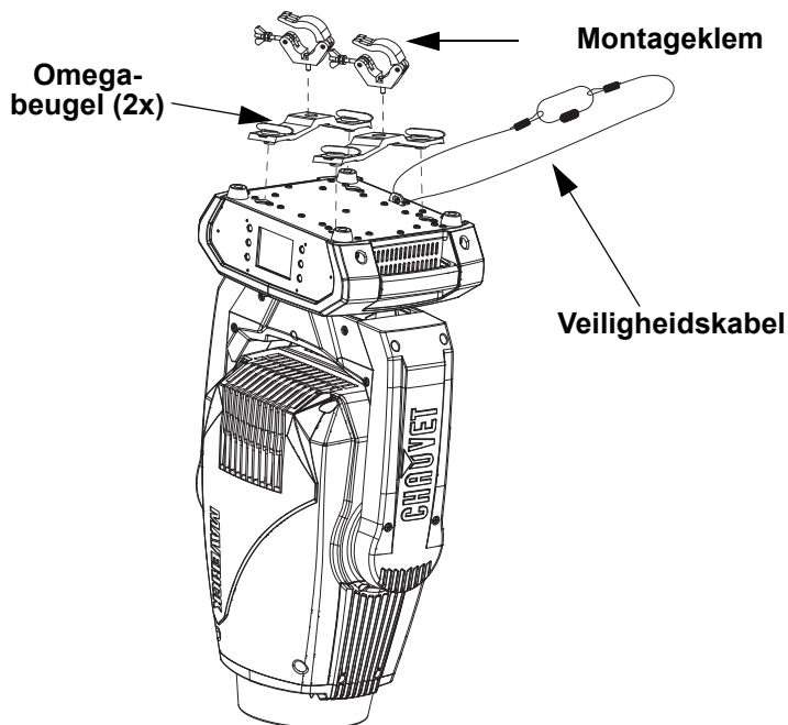
Montage boven het
