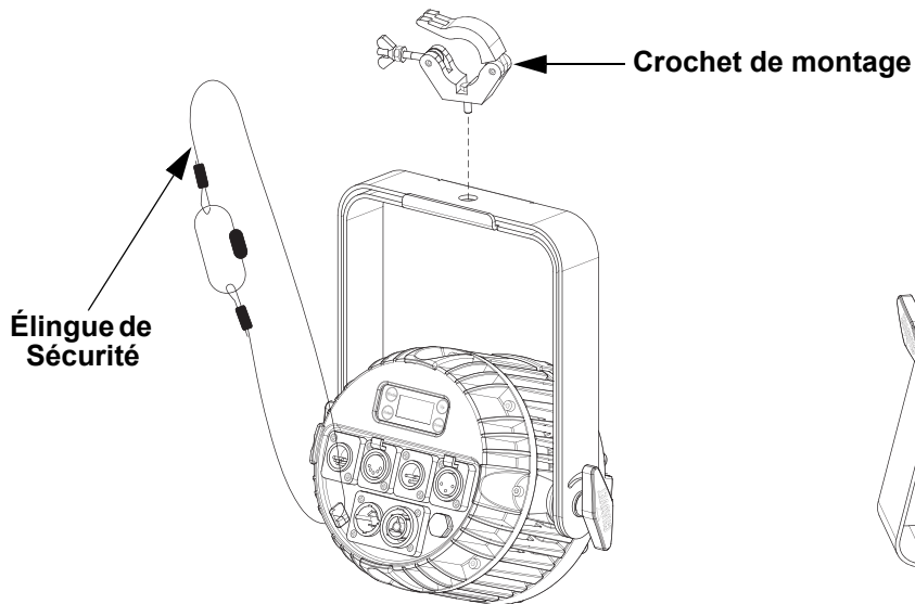
Montage en hauteur
